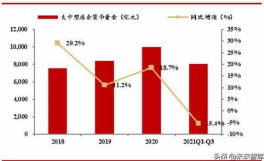
图 33 15 家大中型房企货币资金及变动
